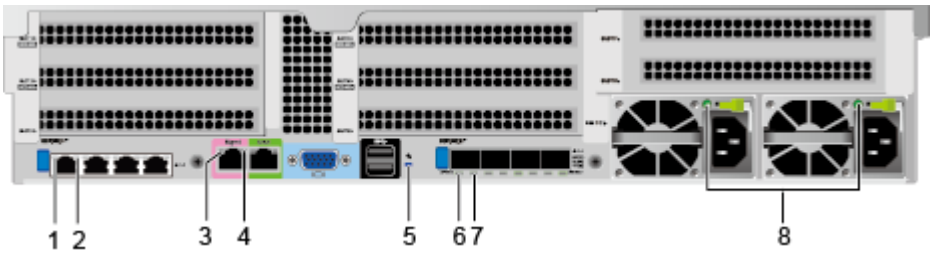
图 4-11 后面板指示灯
