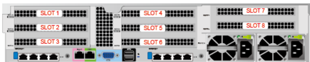
图 4-23 PCIe 插槽
