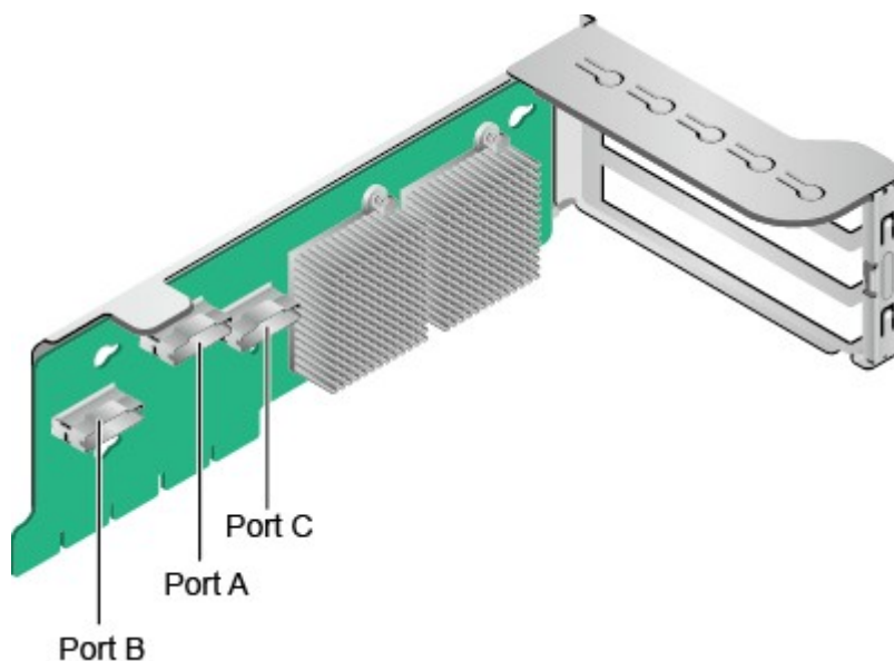
图 4-18 12NVMe 专用 Riser 卡 3（板名：BC82PRUD）
