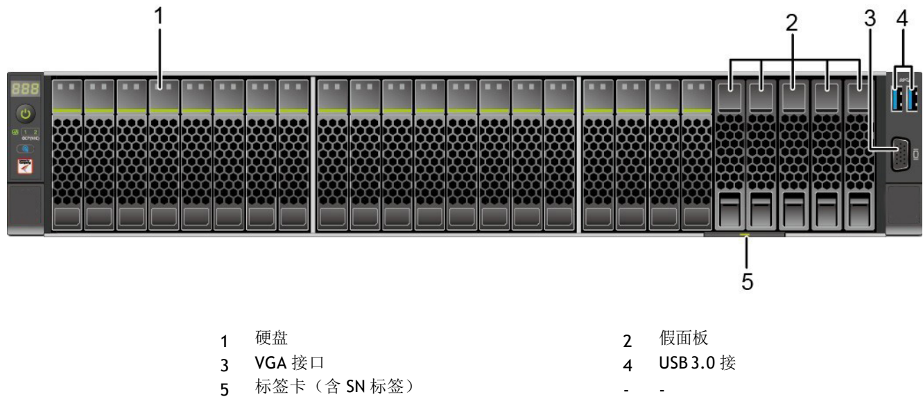
图 4-3 8x2.5 SAS/SATA+12x2.5 NVMe 硬盘配置前面板组件
