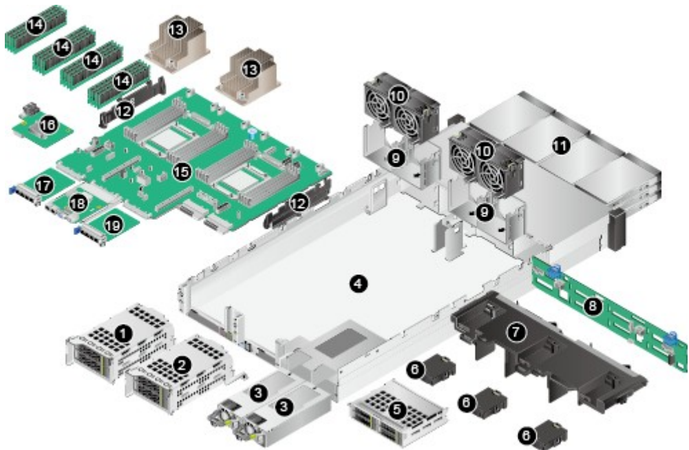
图 4-25 部件（配置鲲鹏 920 5220、5221K、3211K 或 3210 处理器）
