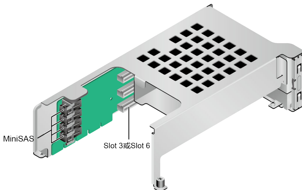
图 4-20 SAS Riser 卡 5（板名：BC82PRNE）
