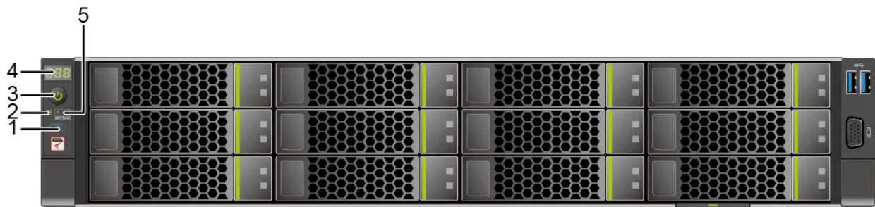
图 4-7 12x3.5 英寸硬盘配置前面板指示灯和按钮
