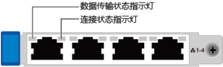
图 4-14 TM210（4*GE 电口）
