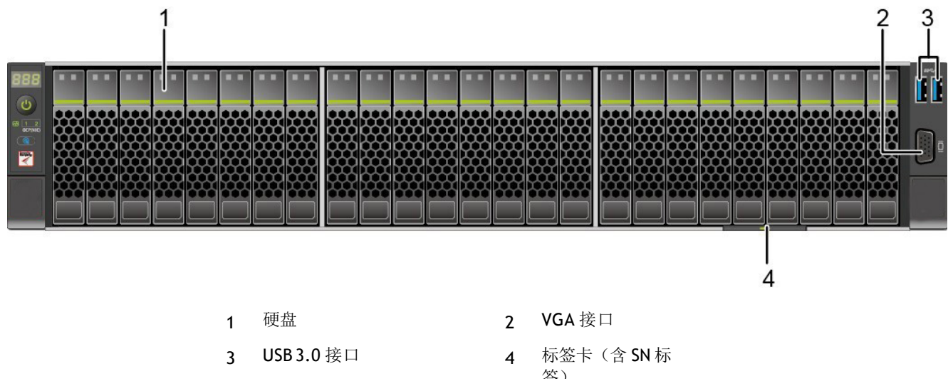
图 4-2 25x2.5 英寸硬盘配置前面板组件
