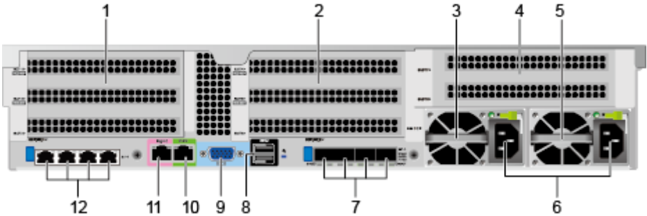
图 4-6 后面板组件
