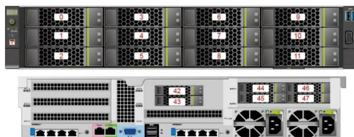
图 6-4 12x3.5 英寸直通硬盘配置
